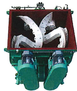
二軸強制練ミキサ
